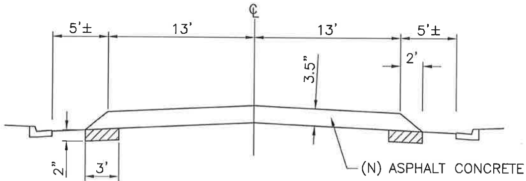
CROSS-SECTION N.T.S.
