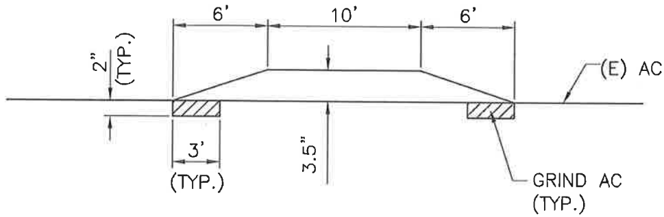
PROFILE N.T.S.
